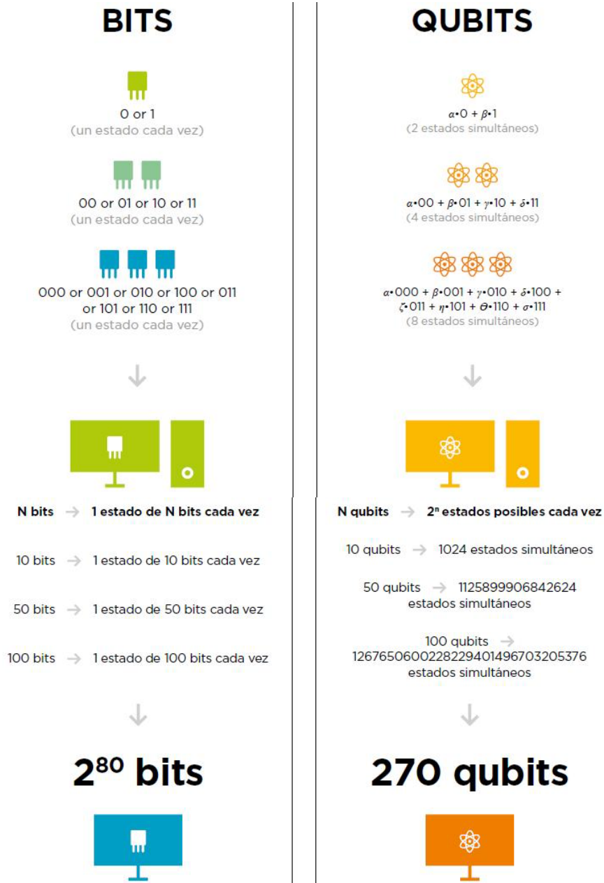
Figura 3. Bits versus Cúbits
