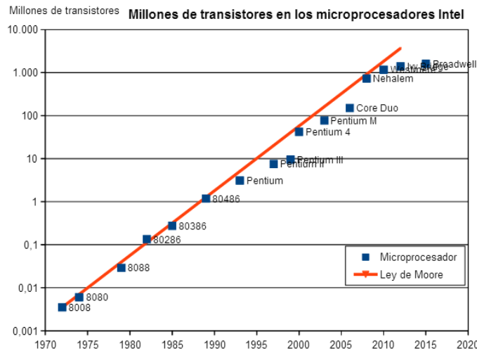
Figura 5. Crecimiento según la Ley de Moore
