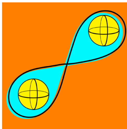
Figura 11. Entrelazamiento cuántico.
