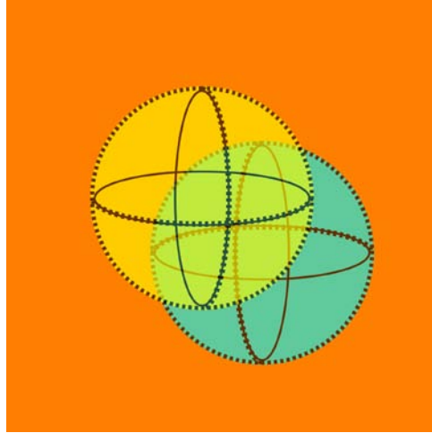
Figura 10. Superposición cuántica.
