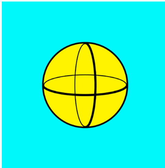
Figura 9. Representación idealizada de un cúbit.
